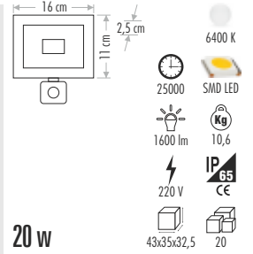
CT-4652 SENSÖRLÜ SLİM LED PROJKTÖR 155,00 ₺
