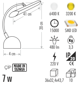
CT-5212 KUĞU LEDLİ APLİK 140,00 ₺
