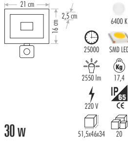
CT-4653 SENSÖRLÜ SLİM LED PROJKTÖR 180,00 ₺
