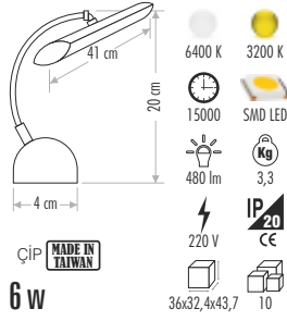
CT-5246 KUĞU LEDLİ APLİK 150,00 ₺
