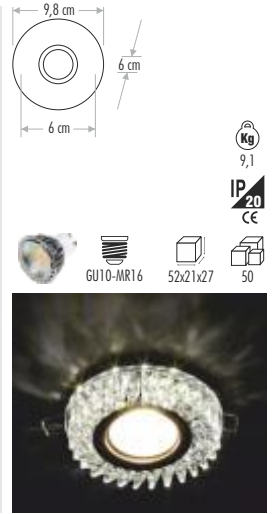
CT-6610 BADEM LED ÇERÇEVELİ (GÜN IŞIĞI) 45,00 ₺
