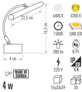
CT-5205 FLAMİNGO LEDLİ APLİK 105,00 ₺
