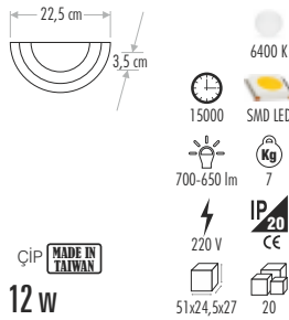
CT-5157 YARIM AY LEDLİ APLİK SIVA ÜSTÜ 75,00 ₺
