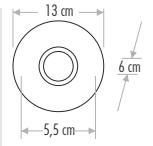
CT-6583 HANİMELİ LED ÇERÇEVELİ (GÜN IŞIĞI) 55,00 ₺
