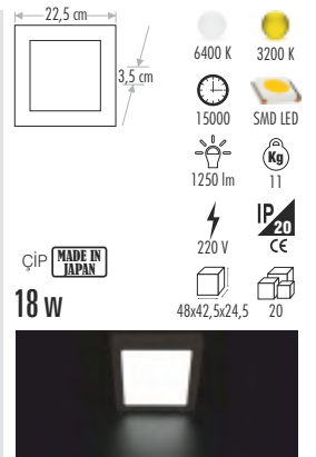
CT-5234 S DAMLA LED ARMATÜR SIVA ÜSTÜ 70,00 ₺
