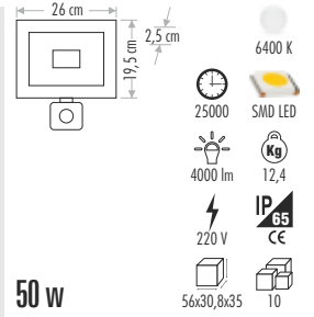
CT-4654 SENSÖRLÜ SLİM LED PROJKTÖR 220,00 ₺
