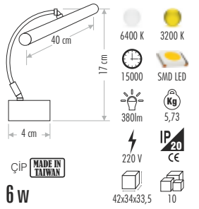
CT-5206 FLAMİNGO LEDLİ APLİK 135,00 ₺
